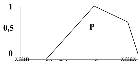
Fig.2 Insieme fuzzy.
